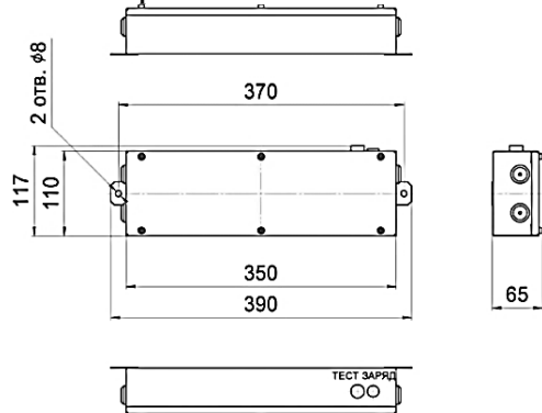
Рис. 10 Блок аварийного питания BS-STABILAR2-81-B2-LED BOX IP65
