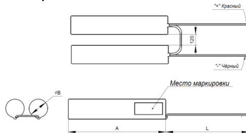
Батарея BS-3+3HRHT14/50-1,6/A-HB500-0-1 a18279
