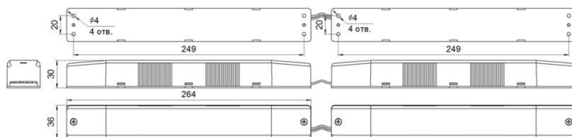
Рис. 10 Блок аварийного питания BS-STABILAR2-81-B2-LED BOX IP65
