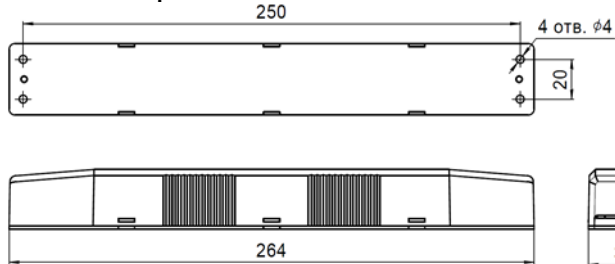
Рис. 7 Блок аварийного питания BS-STABILAR2-81-B2-LED
